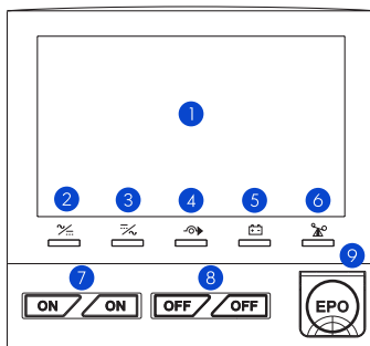
Figura 2-2 Apariencia del Tablero de control del UPS-IND HF 1300 MI
