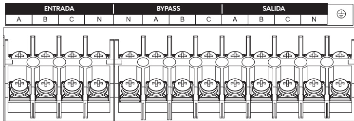
Figura 3-18 Identificadores del terminal de cableado del UPS-IND HF 1300 MI (15-20 kVA)
