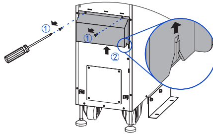
Figura 3-12 Retiro de la cubierta del cableado del UPS-IND HF 1300 MI (10 kVA)
