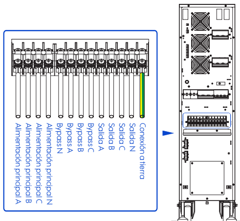
Figura 3-19 Esquema de cableado 1 del UPS-IND HF 1300 MI (15-20 kVA)
