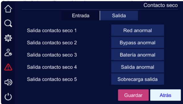
Figura 4-36 Pantalla 1 de configuración de contacto seco de salida
