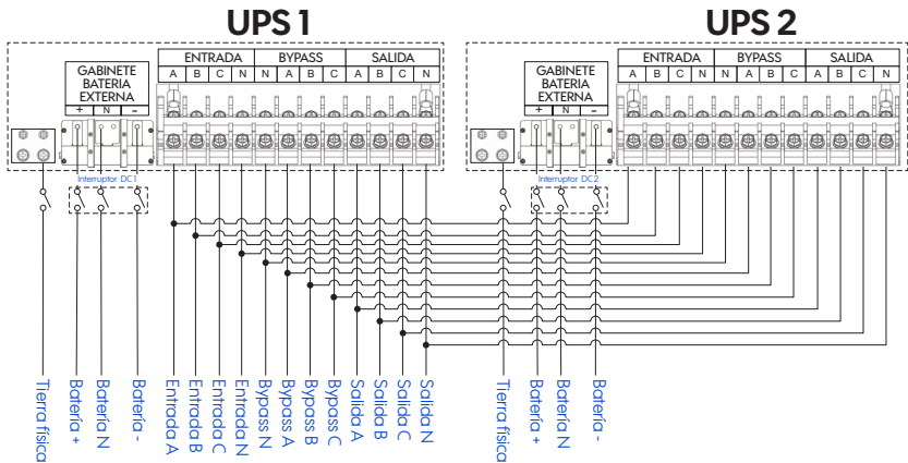
Figura 3-26 Esquema de cableado del sistema en paralelo del UPS-IND HF 1300 MI (30 kVA)
