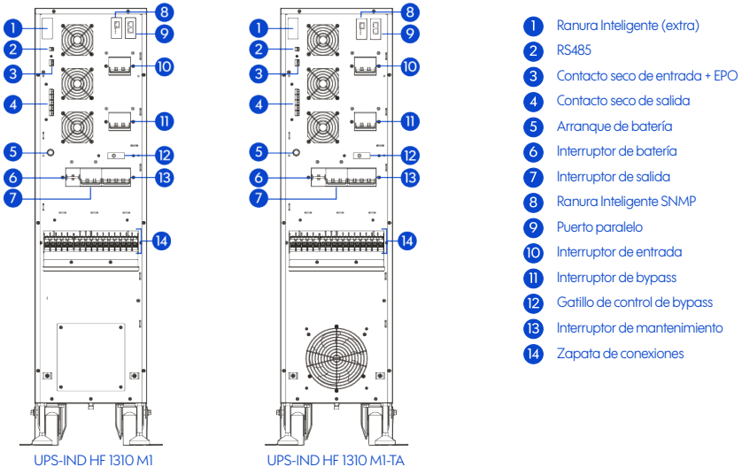
Figura 2-3 Apariencia del panel posterior del UPS-IND HF 1300 MI (10 kVA)
