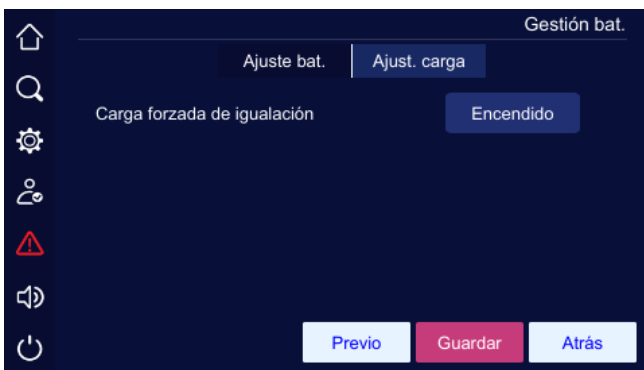
Figura 4-32 Gestión de baterías (pantalla 2 de configuración de carga)
