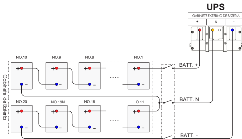
Figura 3-32 Esquema de cableado para UPS-IND HF 1300 MI (30 kVA)
