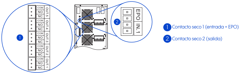
Figura 2-6 Posición de contactos secos del UPS-IND HF 1300 MI
