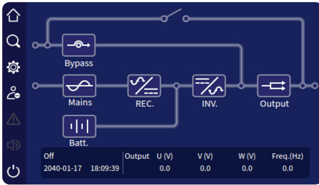
Figura 4-2 Pantalla principal del UPS-IND HF 1300 MI
