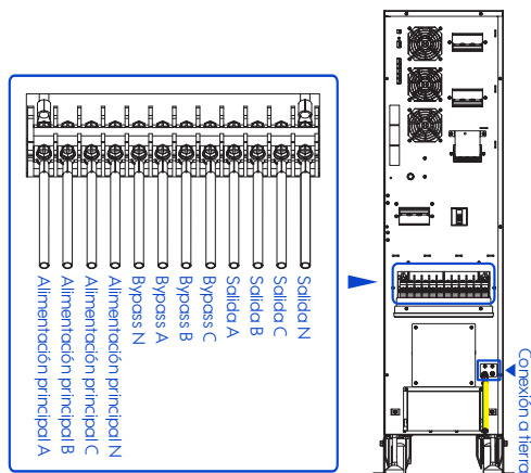
Figura 3-24 Esquema de cableado 1 del UPS-IND HF 1300 MI (30 kVA)
