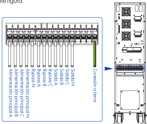
Figura 3-14 Esquema de cableado 1 del UPS-IND HF 1300 MI (10 kVA)
