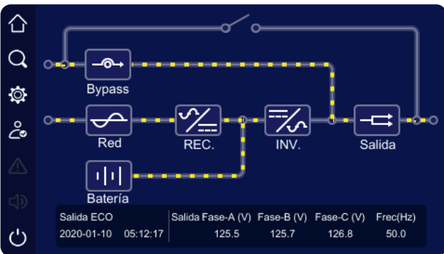
Figura 4-7 Modo ECO
