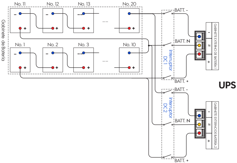
Figura 3-29 Esquema 1 de cableado para UPS-IND HF 1300 MI (15-20 kVA)
