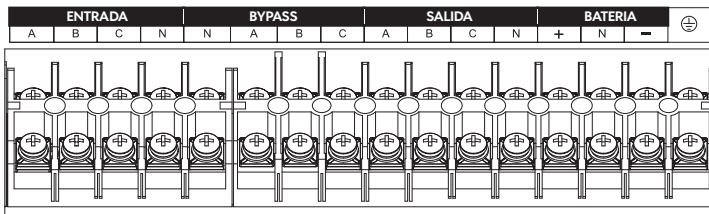
Figura 3-13 Identificadores del terminal de cableado del UPS-IND HF 1300 MI (10 kVA)
