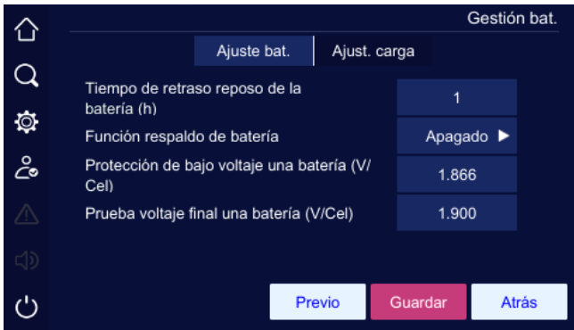
Figura 4-30 Gestión de baterías (pantalla 2 de configuración de batería)
