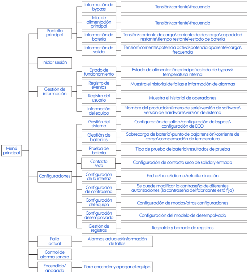
Figura 4-1 Estructura del menú de la pantalla táctil del UPS-IND HF 1300 MI
