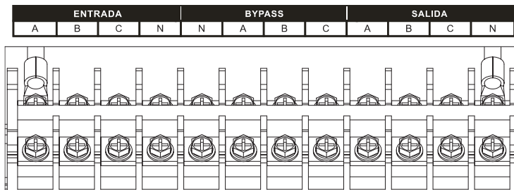
Figura 3-23 Identificadores del terminal de cableado del UPS-IND HF 1300 MI (30 kVA)
