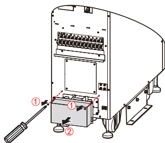
Figura 3-31 Desmante la placa de cubierta
