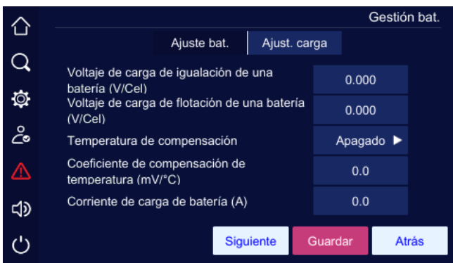
Figura 4-31 Gestión de baterías (pantalla 1 de configuración de carga)
