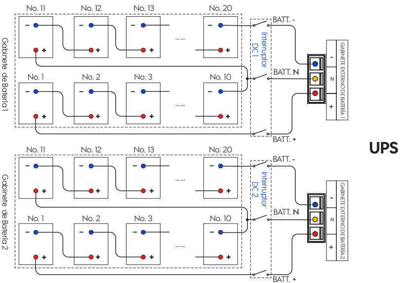
Figura 3-30 Esquema 2 de cableado para UPS-IND HF 1300 MI (15-20 kVA)
