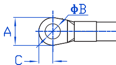
Figura 3-6 Dimensiones del terminal de cableado del UPS-IND HF 1300 MI
